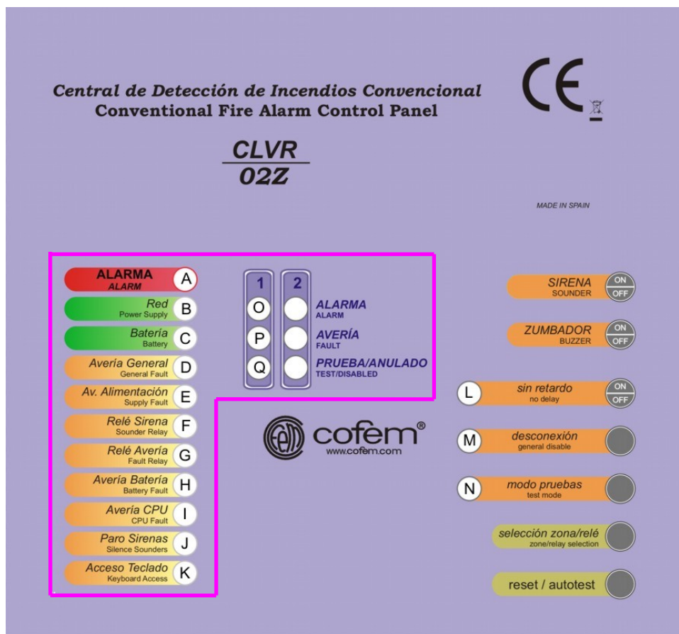
Figura 13: Indicadores utilizados en las pruebas de avería y baterías
