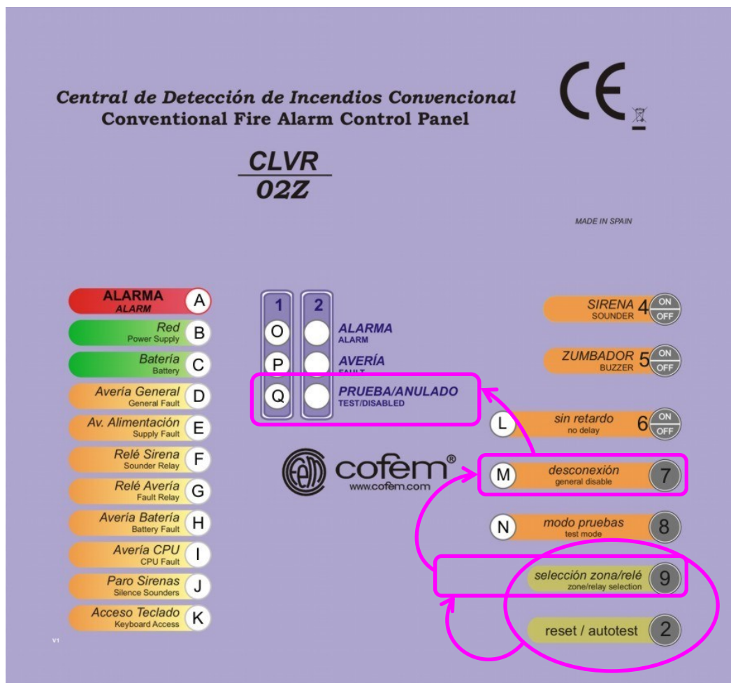
Figura 12: Teclas e indicadores utilizados en la desconexión de zonas
