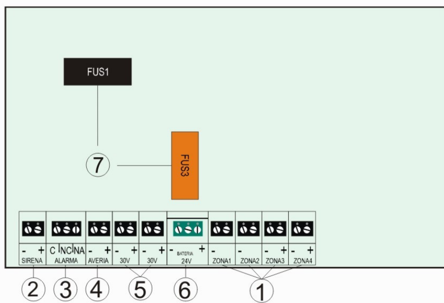
Figura 6: Esquema de los conectores de la central CLVR 02Z
