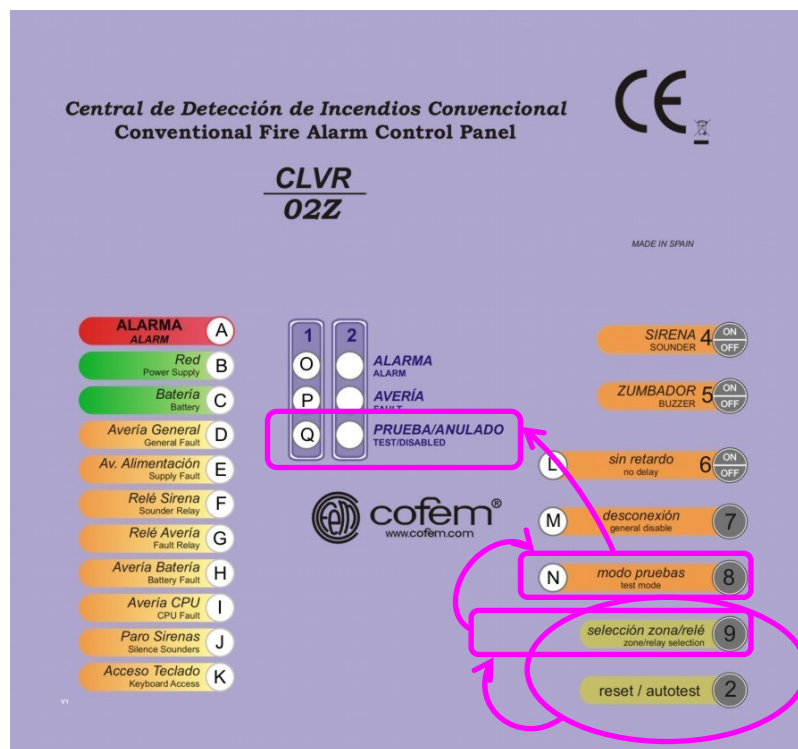
Figura 14: Teclas e indicadores utilizados en las pruebas de los elementos de detección
