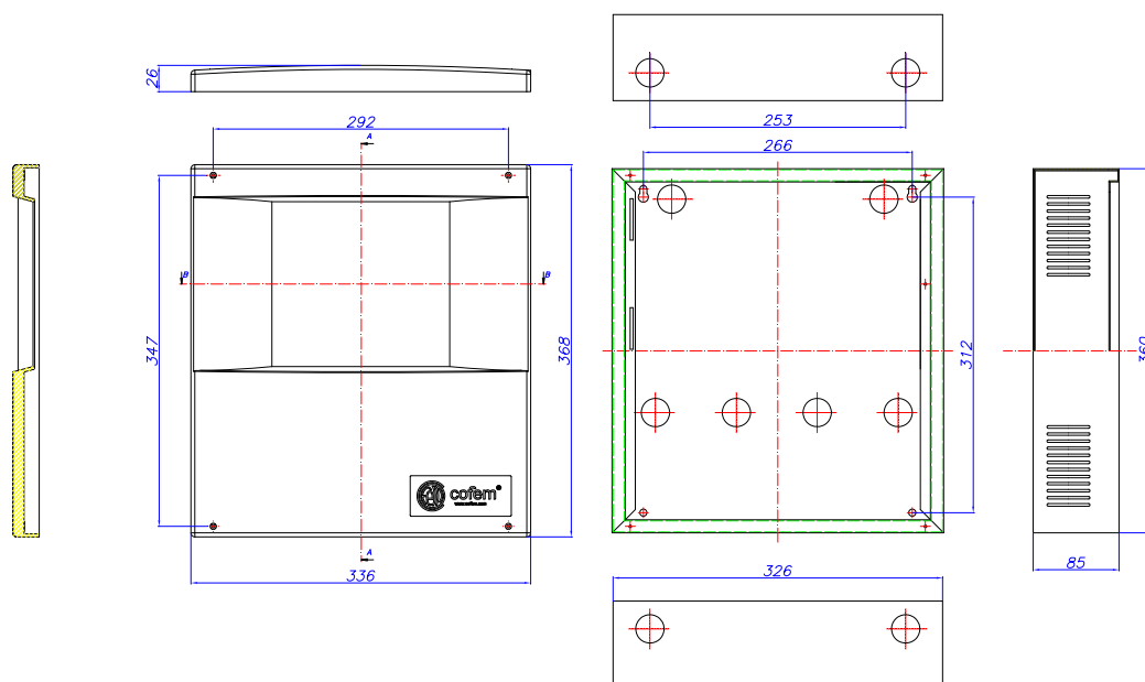
Figura 5: Dimensiones puerta y cofre central (mm).
