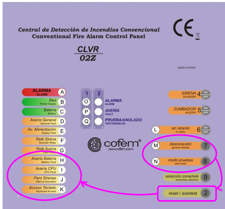
Figura 15: Teclas e Indicadores utilizados en las consultas de versión de software y versión de configuración de retardos.
