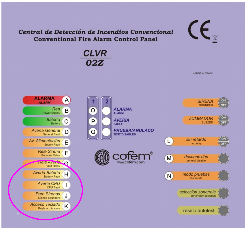
Figura 10: Indicadores luminosos usados para la configuración del tiempo de retardo.
