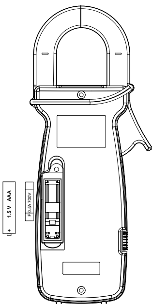
Abb. 4. Batteriesicherung
